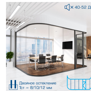
ПРЕМИУМ 82+ РАДИУС ■ Безрамное радиусное остекление с алюминиевым профилем сечением 38*82 мм по периметру; ✓ Max высота = 2800 мм, радиус больше 1100 мм.
