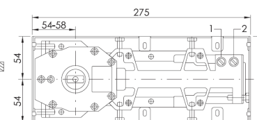
Скрытый напольный доводчик с фиксацией
