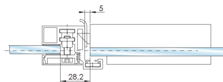
Горизонтальный разрез двери
