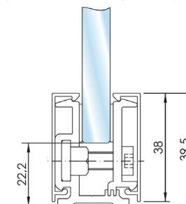
Чертеж зажимной коробки в разрезе
