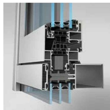
Створка, интегрированная в фасад
