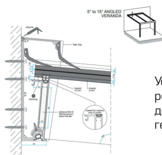
Односкатная крыша с многоугольником с двух сторон
