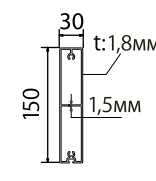
③.1 Профиль под козырек
