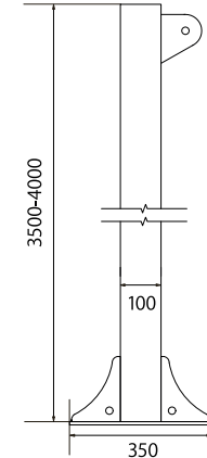
④.2 Балка тента
