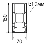
⑤ Жесткий подвес
